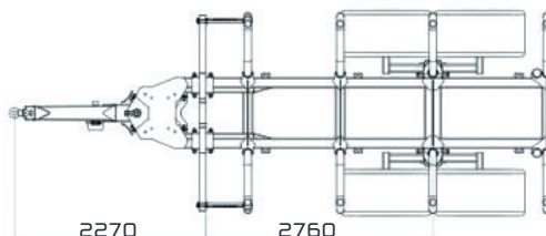
DIMENSIONS
