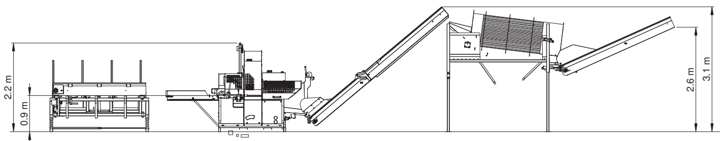
DIMENSIONS
